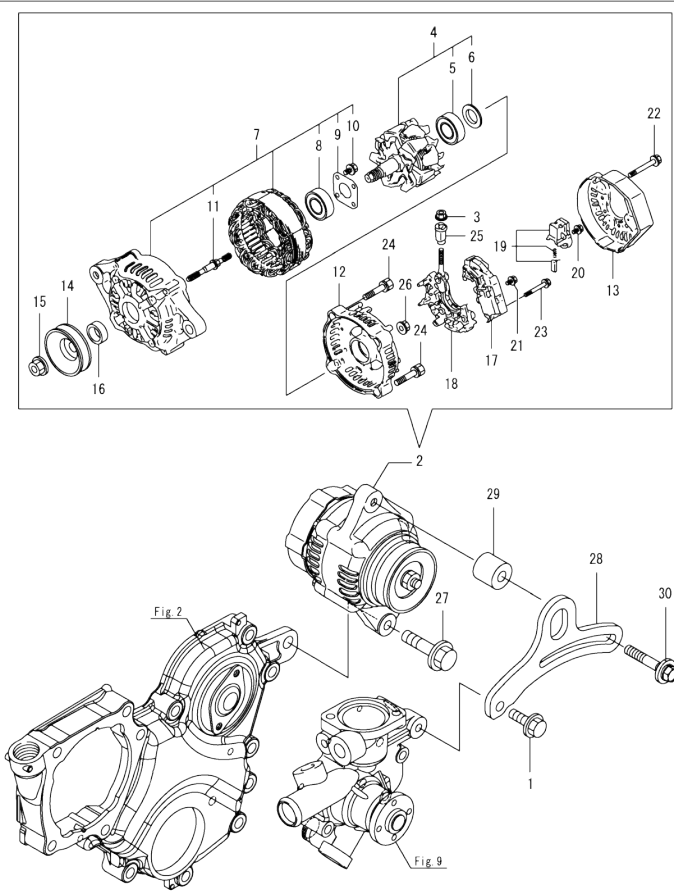
Fig.15. GENERATOR
